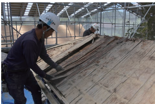
写真4 下地（杉皮）の解体状況（渡廊下東面）
