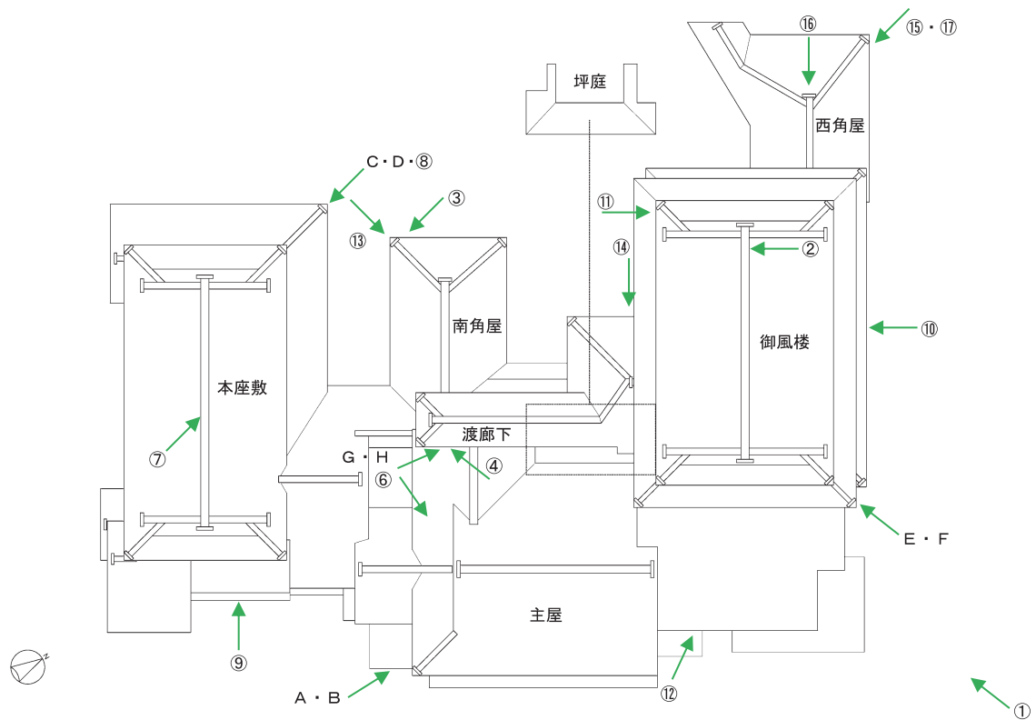
図1 濱口家住宅（主屋・本座敷・御風楼）屋根伏図および写真撮影位置図
