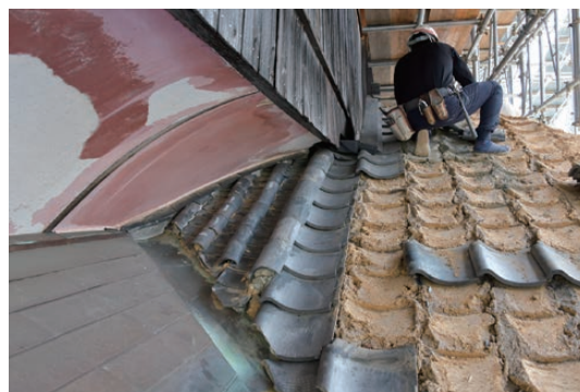
写真14 渡廊下北側三畳 瓦の解体状況 （西より見る）
