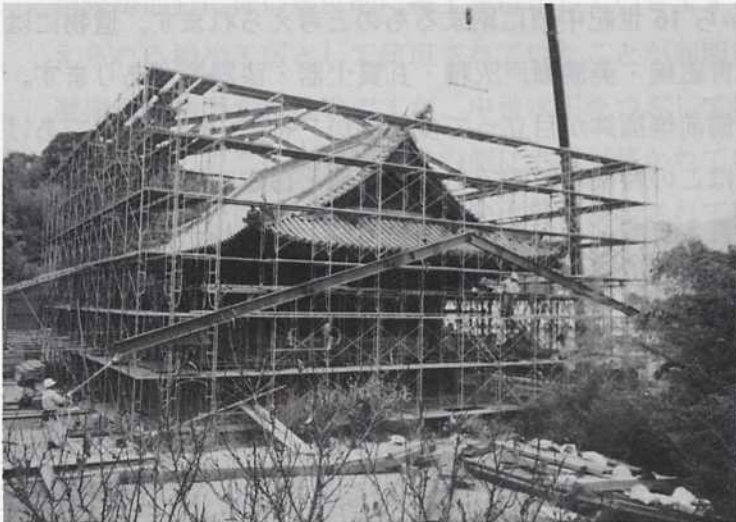
■ 仮設素屋根解体の状況
