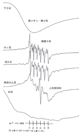
図 2-2-2 産地別滑石・片岩原石の 代表的な E S R スペクトル
