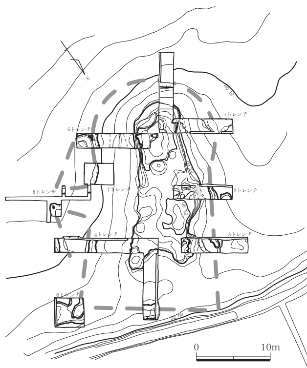
図23 平池1号墳 調査区配置図・平面図
