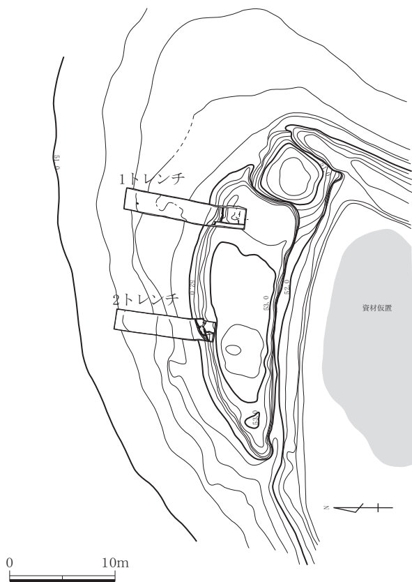
図30 平池4号墳 調査区配置図・平面図・土層図
